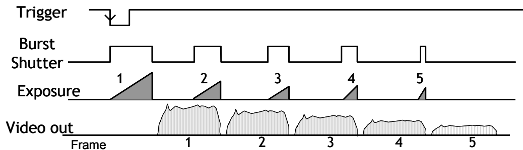
Fig. 9. Burst trigger
